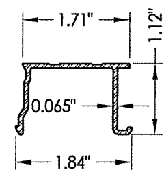
6 SILL CAP 356-A51-52-COV
