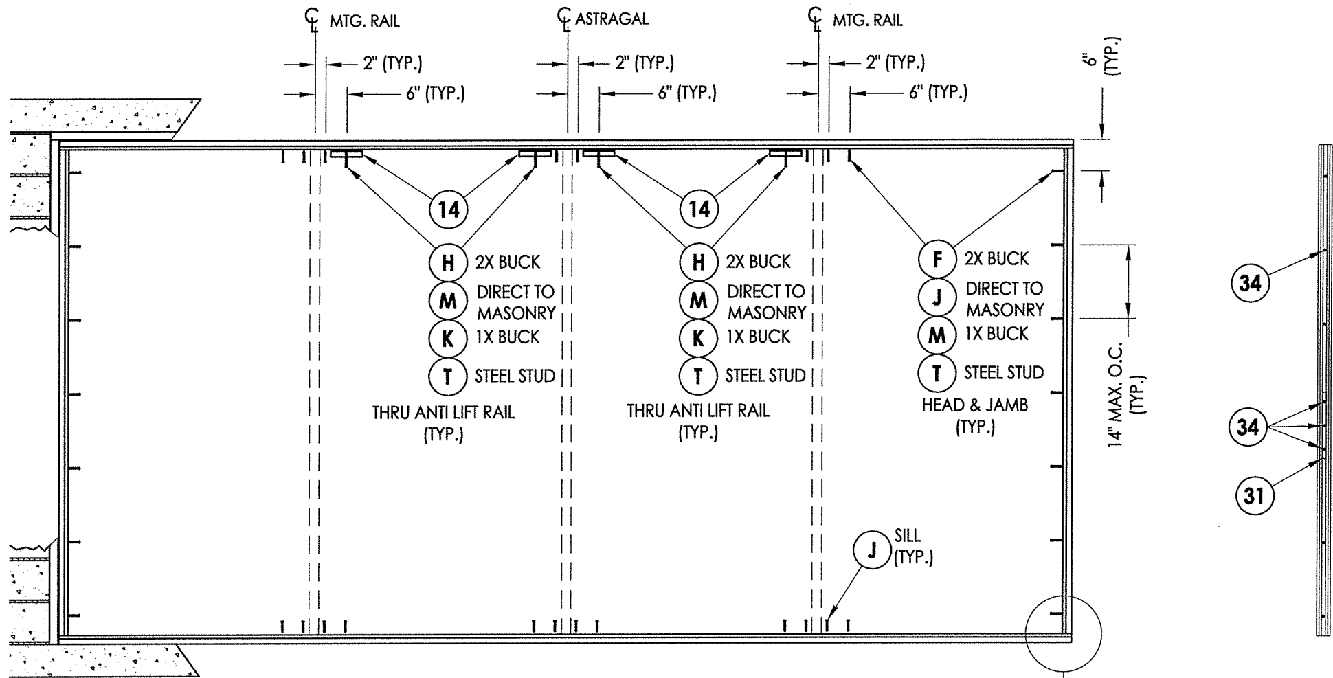
ASTRAGAL
