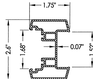
19 ASTRAGAL
