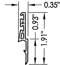
21 SILL RISER
